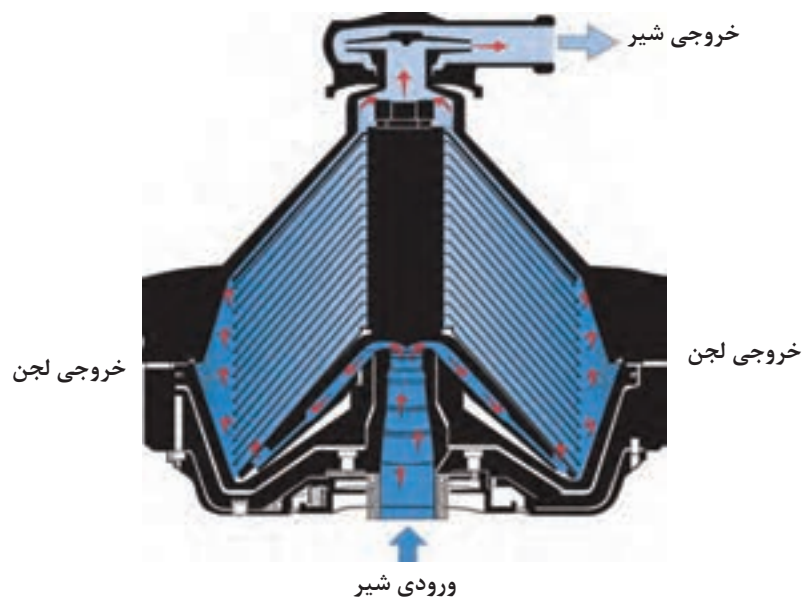
شکل ۱-۱۰- کلاریفایر
