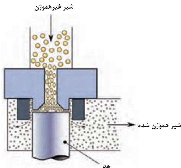
شکل ۲-۴- اصول کار هموژنیزاسیون
