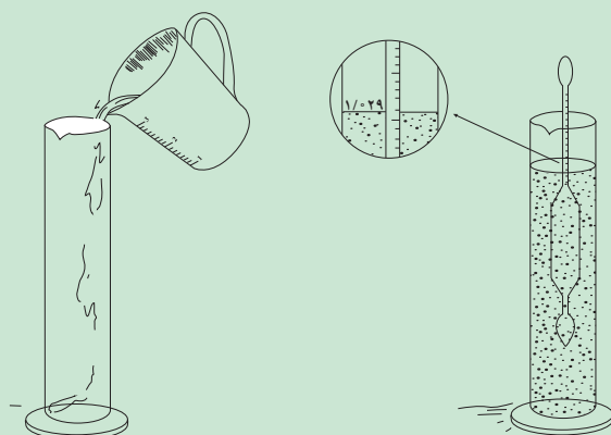
شکل ۱-۷- اندازه‌گیری چگالی با لاکتودانسیومتر
