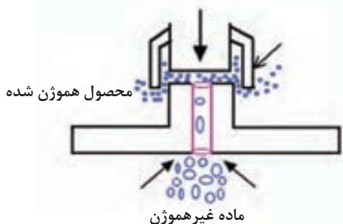
شکل ۱۳-۱- هموژنایز دو مرحله‌ای و تک مرحله‌ای
