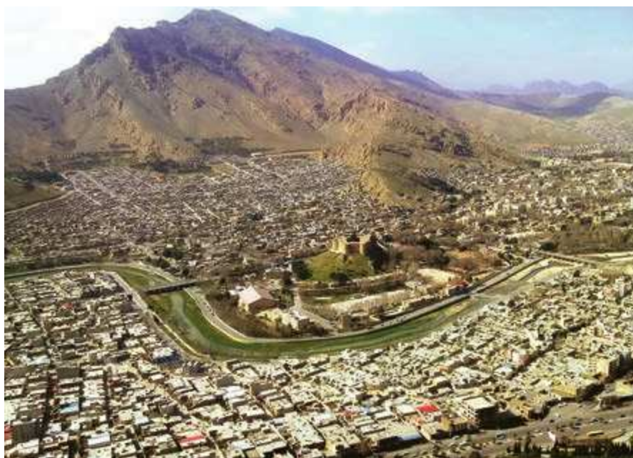
شکل ۹- تغییر در مجرای رود خرم آباد - لرستان
