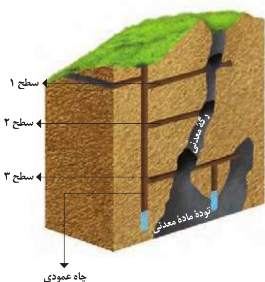
شکل ۹-۲- نحوه بهره برداری از معادن زیرزمینی
