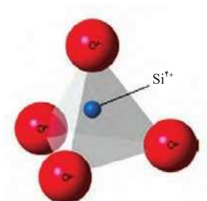
شکل ۲-۱. از اتصال چهار اتم اکسیژن به یک اتم سیلیسیم، هرم چهاروجهی تشکیل می‌شود که واحد بنیادی سیلیکات‌ها است.
