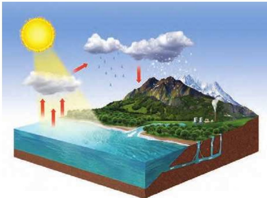
ب) چرخه آب
