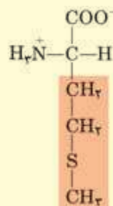
متیونین (Met)
