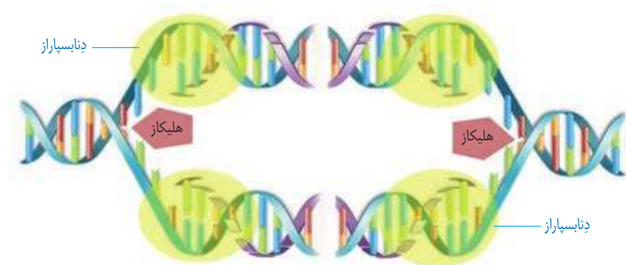
شکل ۱۱- همانندسازی دنا
