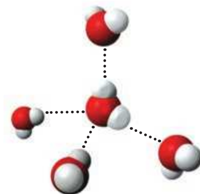
شکل ۱۷- پیوند هیدروژنی میان مولکول‌های \text{H}_2\text{O}
