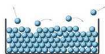
شکل ۴-۲۳ در حین تبخیر سطحی، مولکول‌های پراورزی‌تر از سطح مایع می‌گریزند.
