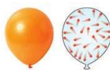
شکل ۲-۶ حرکت نامنظم ذرات گاز درون یک بادکنک
