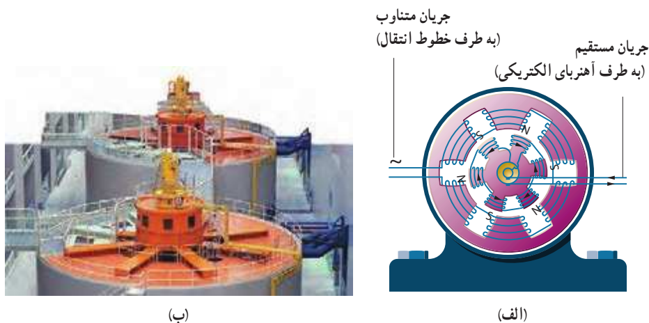
شکل ۱۷-۴ الف) در مولدهای صنعتی با چرخیدن آهنربای الکتریکی بین پیچ‌ها، جریان متناوب تولید می‌شود. ب) نمایی از مولدهای صنعتی تولید برق.
