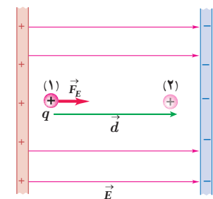
شکل ۲۵-۱ نسبت تغییر انرژی پتانسیل به بار، مستقل از نوع و اندازه بار الکتریکی است.
