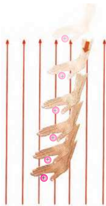
شکل ۲۷-۱ نیروی خارجی، بار +q را در خلاف جهت میدان الکتریکی جابه‌جا می‌کند.
