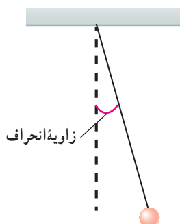
شکل ۳-۸ آونگ ساده، شامل وزنه‌ای کوچک است که از نخ بدون جرم و کش نیامدنی آویزان است.
