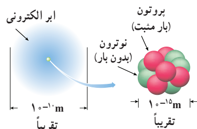
شکل ۴-۲ مقایسه ابعاد اتم و هسته به طور تقریبی
