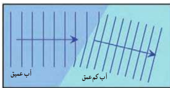
شکل ۳-۴۱ الف) طرحی از شکست امواج سطحی در مرز آب عمیق و آب کم عمق در تشت موج و ب) تصویری واقعی از شکست امواج سطحی در تشت موج
