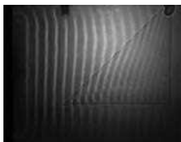
شکل ۳-۴۱ الف) طرحی از شکست امواج سطحی در مرز آب عمیق و آب کم عمق در تشت موج و ب) تصویری واقعی از شکست امواج سطحی در تشت موج
