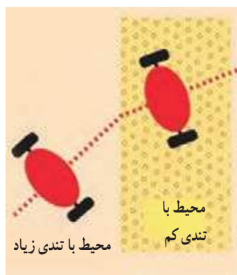
شکل ۱۴-۱۳ وقتی اسباب‌بازی وارد قالیچه می‌شود مسیرش تغییر می‌کند؛ زیرا چرخ‌ها که نخست به قالیچه می‌رسد، زودتر کند می‌شود.
