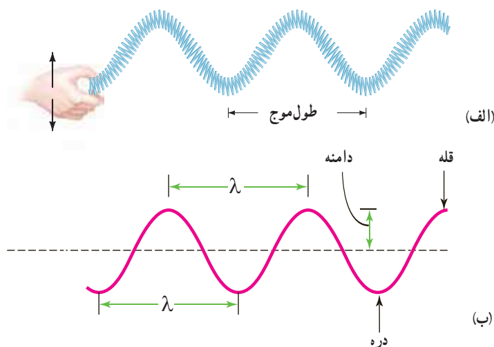
شکل ۳-۱۸ الف) یک موج عرضی در سرفر کشیده شده و ب) مدل سینوسی برای این موج
