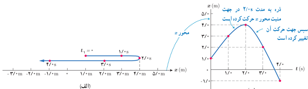
شکل ۱-۴ (الف) مسیر حرکت ذره در امتداد محور x . (ب) نمودار مکان - زمان متحرک
